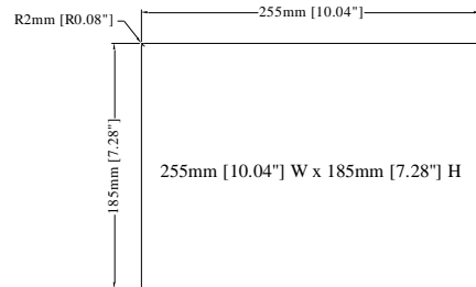
Cutout Dimensions
